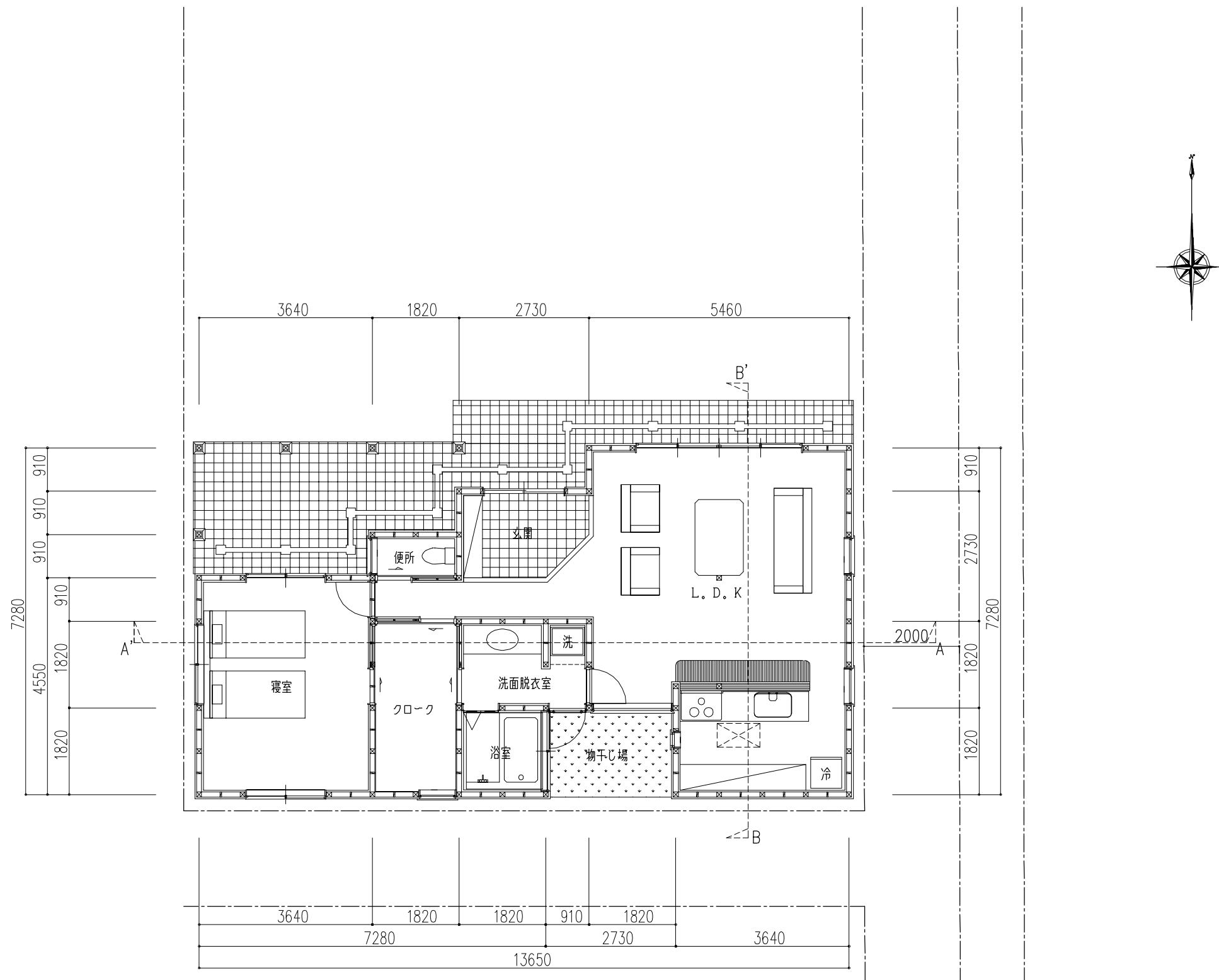
1階平面図 1:100
